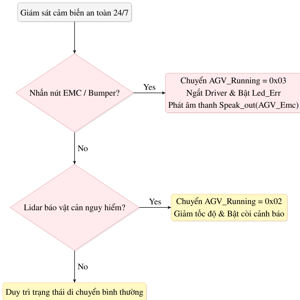
Hình 4.4 Sơ đồ luồng xử lý an toàn Lidar, Bumper và Nút khẩn cấp.
