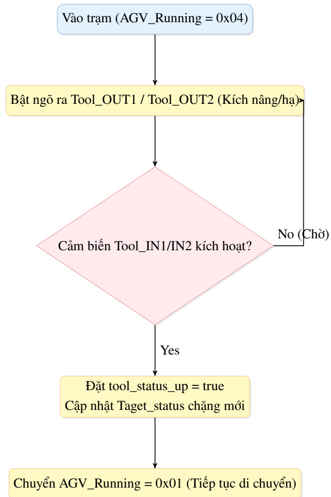
Hình 4.5 Sơ đồ luồng quy trình nâng/hạ móc kéo hàng tự động.
