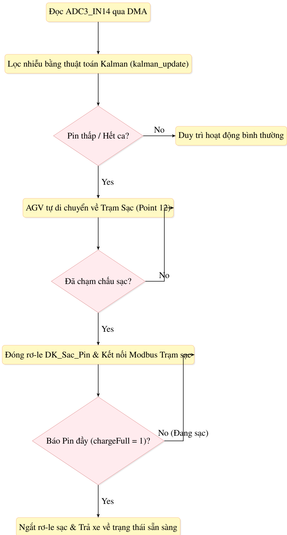
Hình 4.6 Sơ đồ luồng đo điện áp pin Kalman và chu trình sạc tự động.
